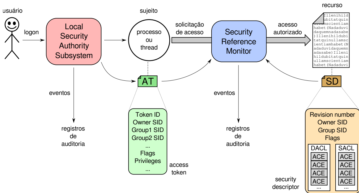
Figura 29.7: Listas de controle de acesso no Windows.
