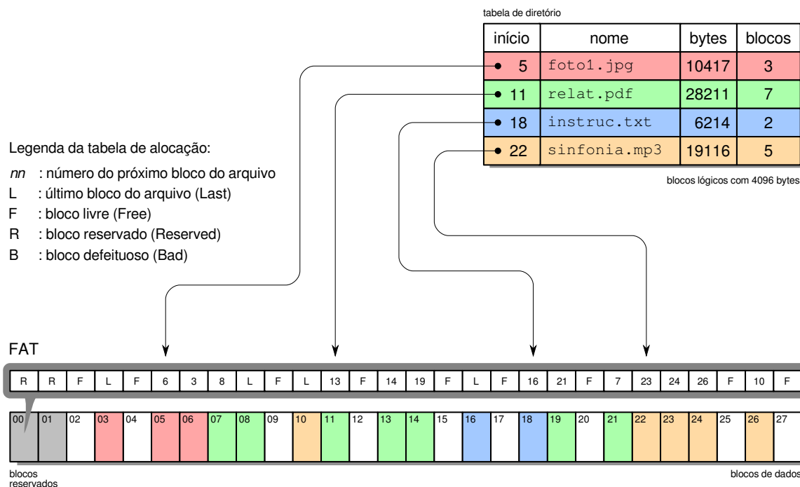
Figura 24.8: Estratégia de alocação encadeada com FAT.
