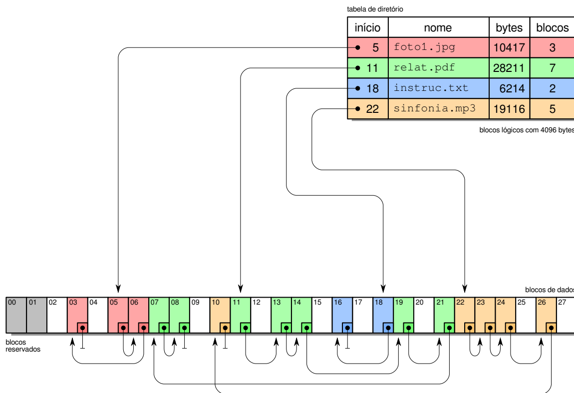
Figura 24.7: Estratégia de alocação encadeada simples.
